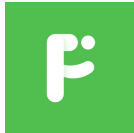
Finnhub API
